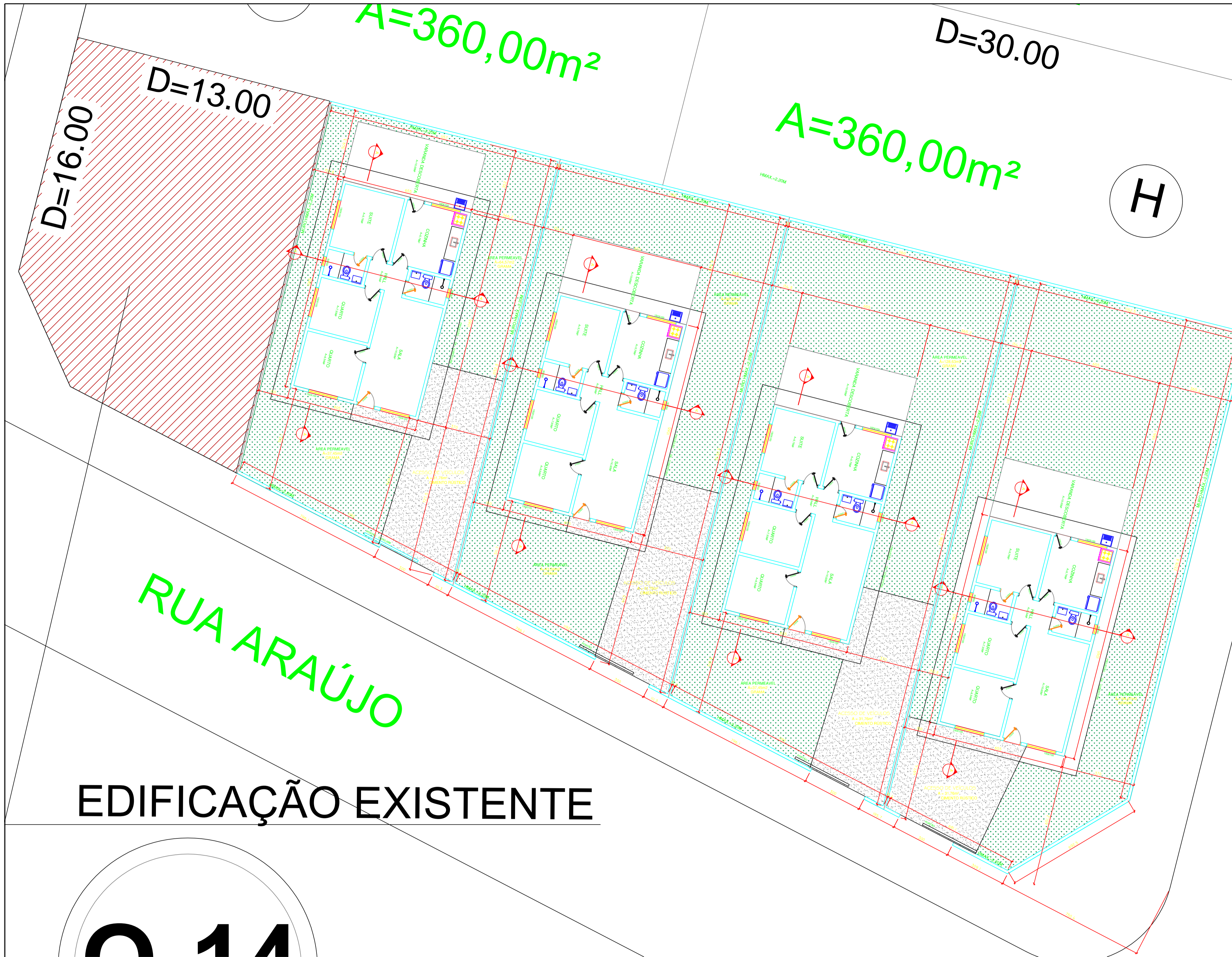
PLANTA - PAV. TÉRREO/LOCAÇÃO ESC. 1:100
